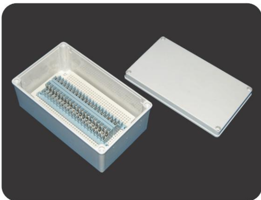
型號(Model): DS-AG-40P-S 尺寸(Size): 150×250×100mm
