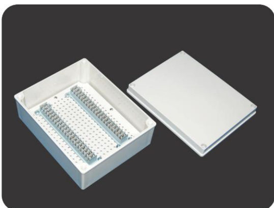
型號(Model): DS-AG-40P-M 尺寸(Size): 200×250×100mm
