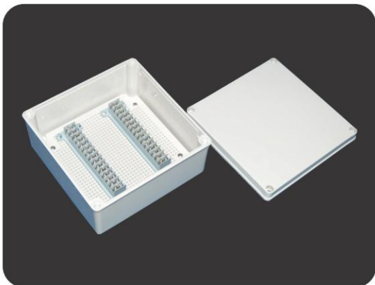
型號(Model): DS-AG-30P-M 尺寸(Size): 200×200×95mm
