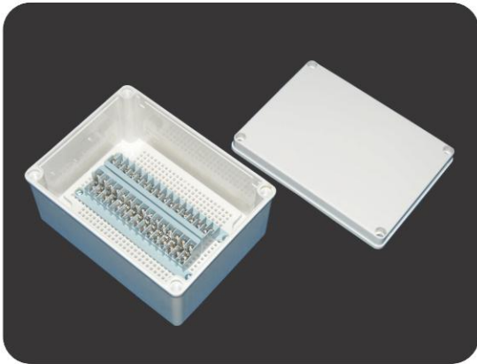
型號(Model): DS-AG-30P-S 尺寸(Size): 150×200×100mm
